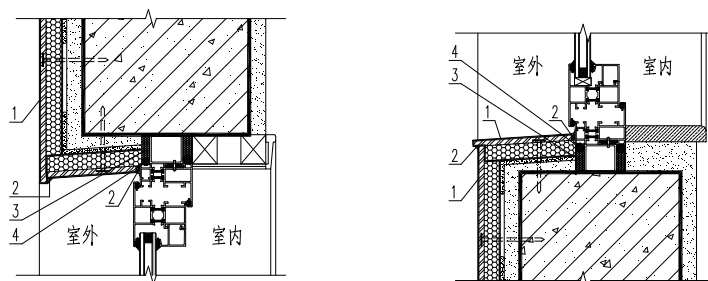
1-保温装饰板；2-硅酮建筑密封胶；3-填缝剂；4-背衬材料
