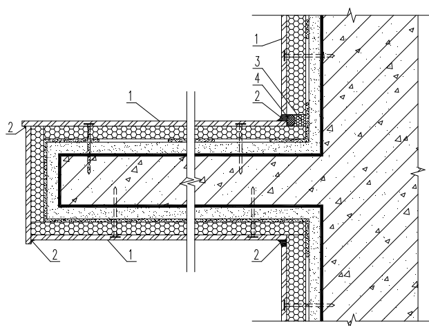
1-保温装饰板；2-硅酮建筑密封胶；3-填缝剂；4-背衬材料
